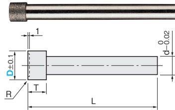
B形状 (側面・底部加工用)
