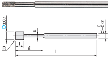
A形状 (側面加工用)
